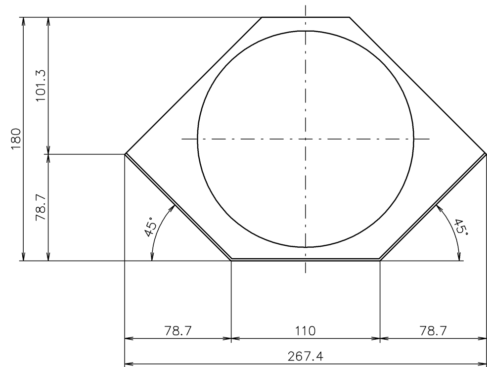
A矢視図
